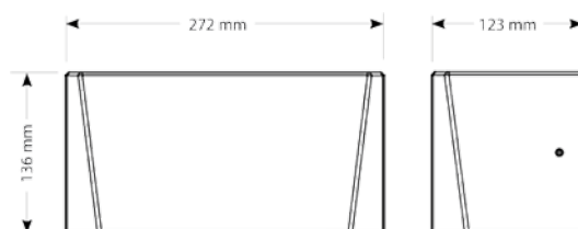
ROZMERY SUŠIČA R4.1
